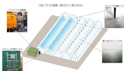
ハウス内自動噴霧装置
